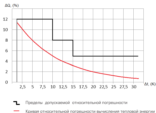
График относительной погрешности вычисления количества тепловой энергии [кВтч], при разности между средней температурой отопительного прибора и температурой воздуха \Delta t , К
